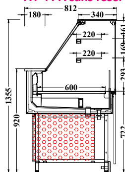
Plan chaud ventilé H1355 AV VPA sans réserve
