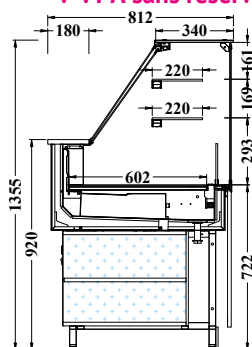
Froid ventilé H1355 V VPA sans réserve
