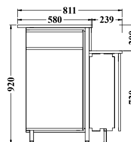
Caisse 2 NIV CX2N
