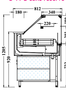
Salad'bar H1205 S VPB sans réserve
