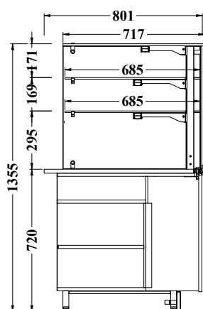
Tours H1355 TV VPA Tour Viennoiserie
