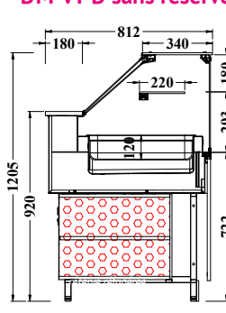
Chaud bain-marie H1205 BM VPB sans réserve
