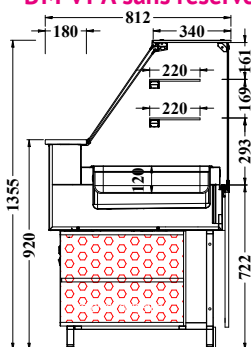
Chaud bain-marie H1355 BM VPA sans réserve
