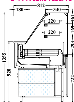
Salad'bar H1355 S VPA sans réserve
