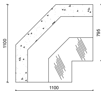
Angles froid ventilé AIR 90 Angle pans coupés 90°int
