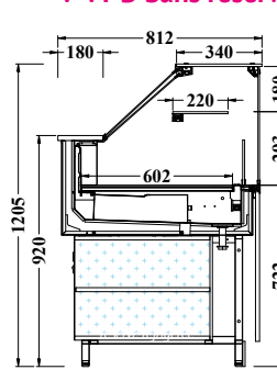
Froid ventilé H1205 V VPB Sans réserve
