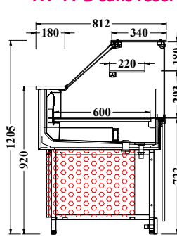
Plan chaud ventilé H1205 AV VPB sans réserve
